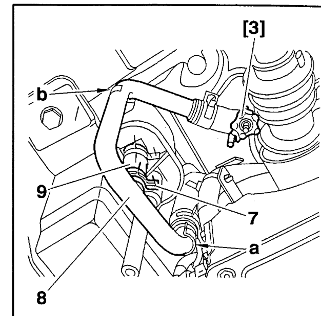
Fig : D1CP00TC Poser l'outil [3]. Déposer le collier (7) ; utiliser l'outil [1]. Dégraffer le tube (8), en "a" et "b". Désaccoupler le tube (8) de la durit (9).
