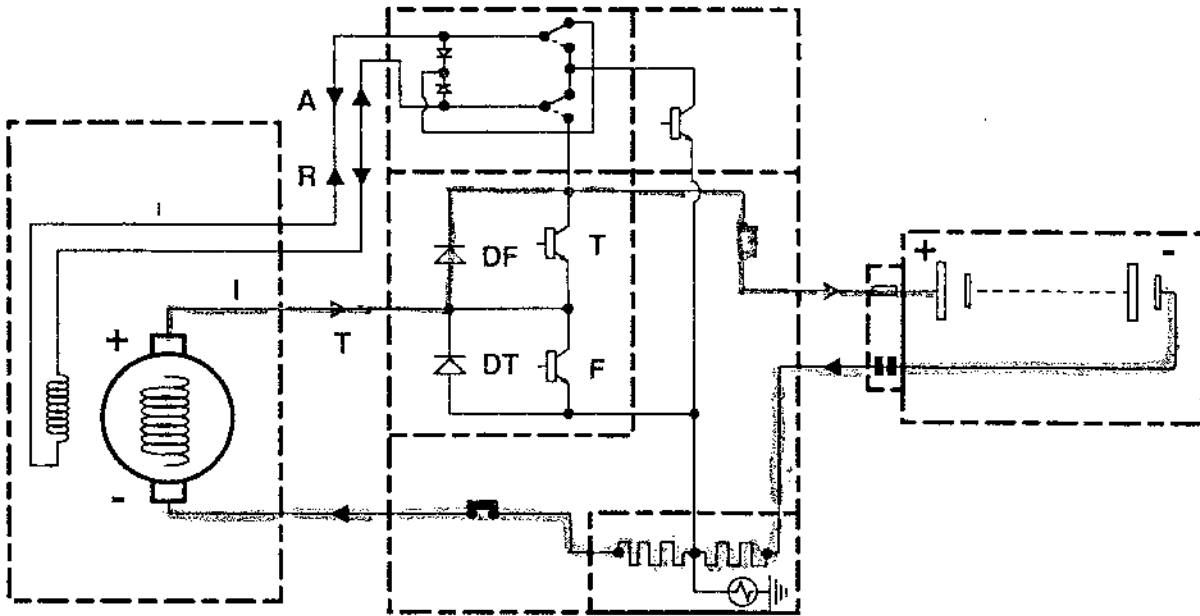
Courant d'induit
